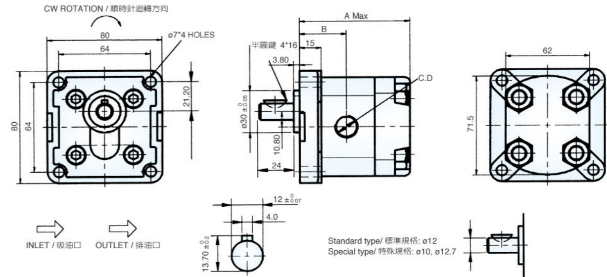
HGP-1A-F*-**-4BE-10 (European / 歐規 4-bolt / 孔式)
