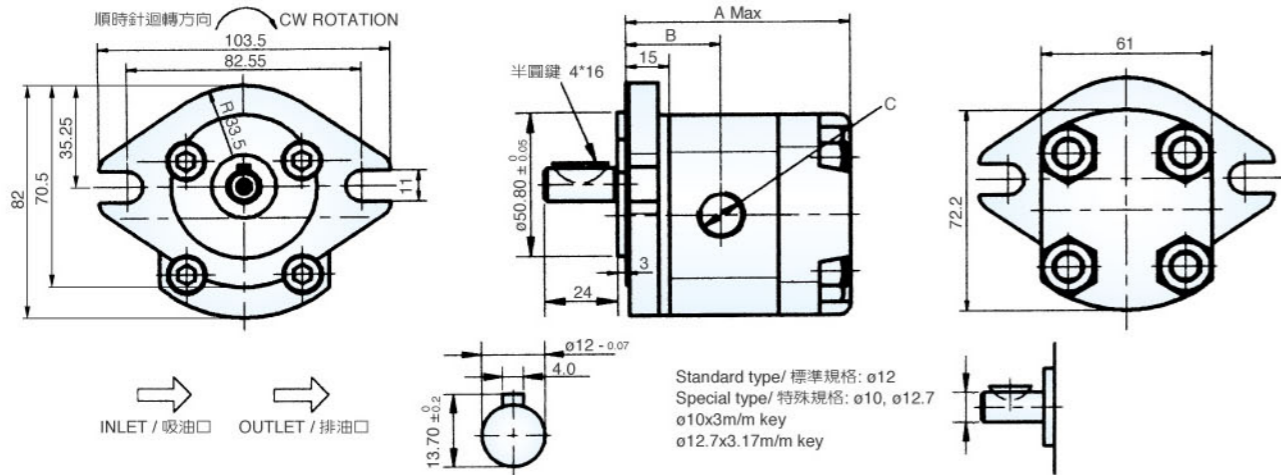
HGP-1A-F*-**-2B-10 (SAE 2-bolt / 孔式)
